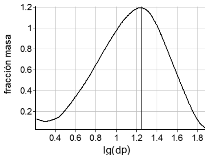
Fig. 7: Distribución del grado de polimerización (dp) de fructanos de agave en formato lineal: Parámetros moleculares calculados: m_{dpw}=18 y m_{dpn}=10 , polidispersidad es m_{(dpw/dpn)}=1.8 .
