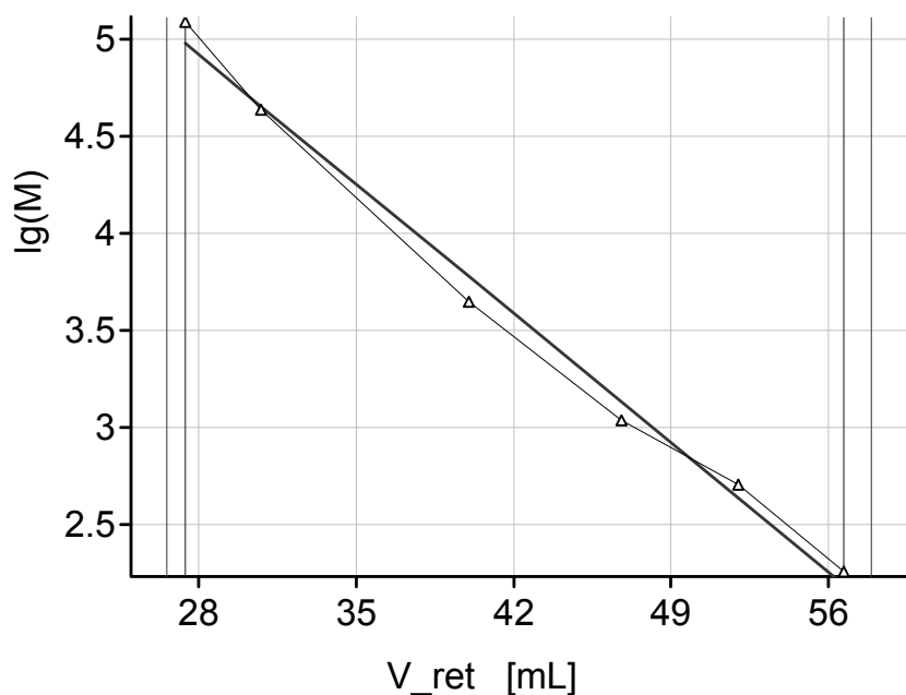
Figura 2: Calibración del sistema SEC con estándares 1 y 2 (puntos triangulares, valores de los picos máximos) y su curva de ajuste lineal (fit_MWV)
