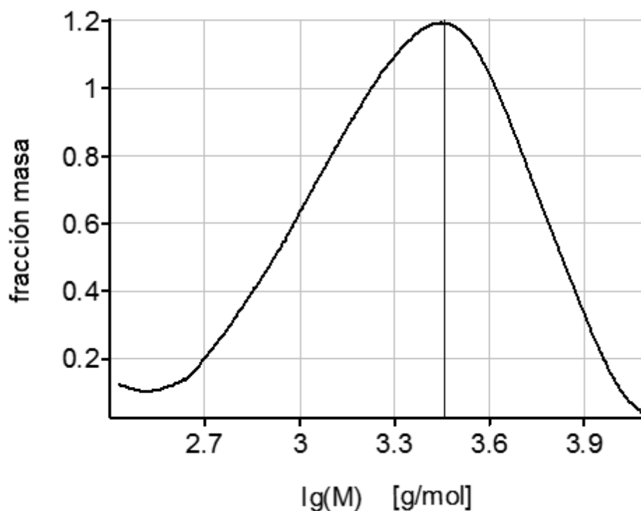
Fig. 5: Distribución de masa molecular (MW) de fructanos de agave en formato logarítmico: Parámetros moleculares calculados: m_{Mw} = 2870 [g/mol] y m_{Mn} =1640 [g/mol], polidispersidad es m_{(Mw/Mn)} =1.75.
