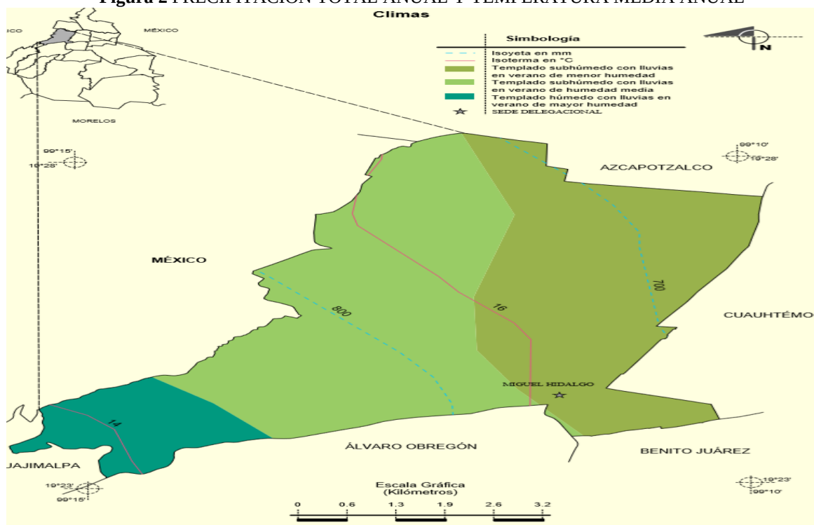
Figura 2 PRECIPITACIÓN TOTAL ANUAL Y TEMPERATURA MEDIA ANUAL
