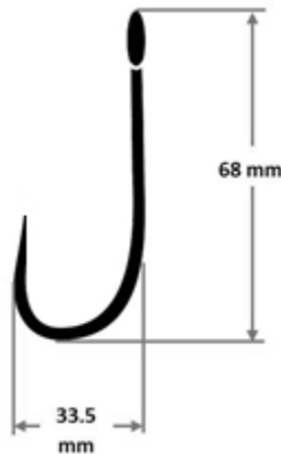
Fig. Dimensiones mínimas de anzuelos atuneros
