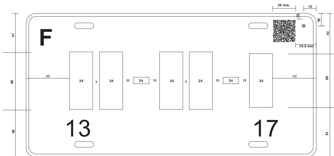
Acotaciones en milímetros El ancho de los caracteres debe ser de acuerdo a lo indicado en la figura Se incorpora la letra "T" y "F" según corresponda a la placa Las dimensiones del guión separador serán de 16 x 5.6 Figura 12 Separación de caracteres (letras y dígitos) placas con cinco caracteres y guiones Placa para DEMOSTRACIÓN (Distrito Federal)
