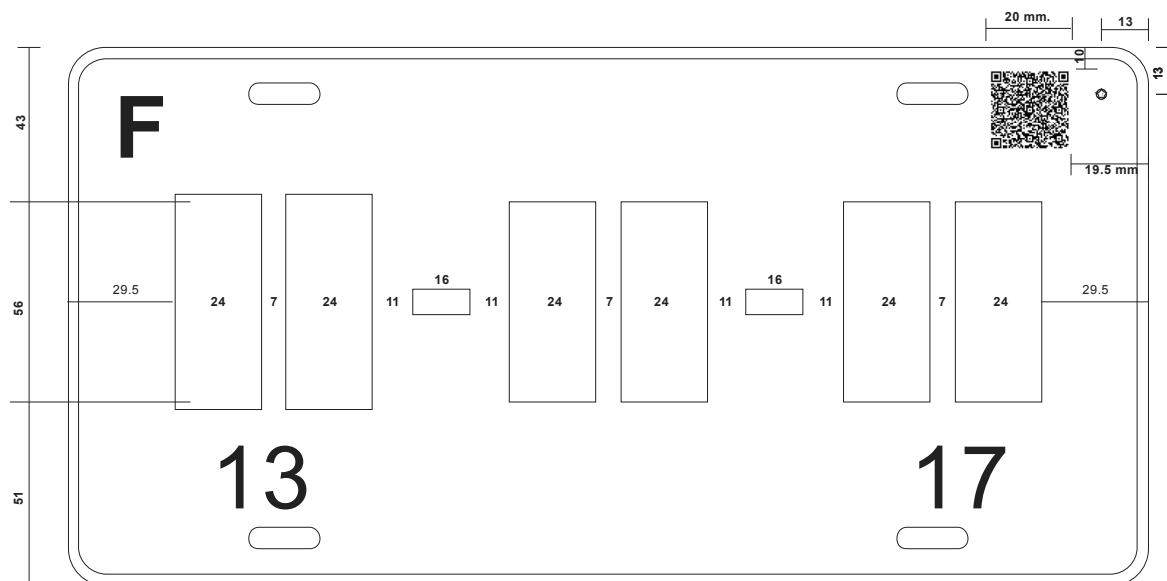
Figura 33 Separación de caracteres (letras y dígitos) placa con seis caracteres y guiones Placa para vehículos del H. CUERPO DE BOMBEROS del Distrito Federal
