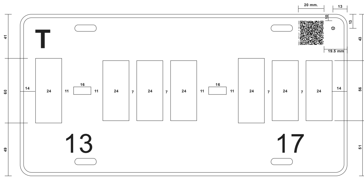
Figura 28 Separación de caracteres (letras y dígitos) placas con siete caracteres y guiones Placa para Remolque Público Local (Entidades Federativas)
