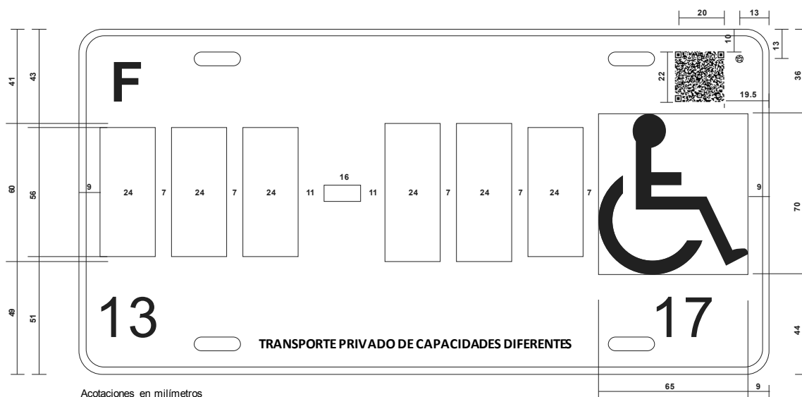
Figura 30 Separación de caracteres (letras y dígitos) placas con seis caracteres y guiones
