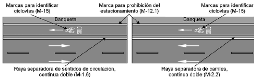
FIGURA 24.- Marcas para delimitar ciclovías
