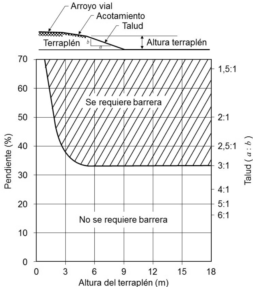
FIGURA 2.- Instalación de barreras de orilla de corona (OD-4.1) en terraplenes (Fuente: Roadside Design Guide AASHTO, USA 2002)
