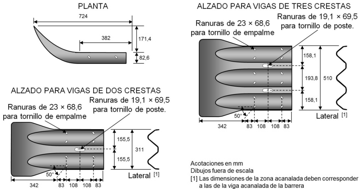
FIGURA 28.- Secciones terminales sencillas para vigas acanaladas de dos y de tres crestas (OD-4.4.2/S)
