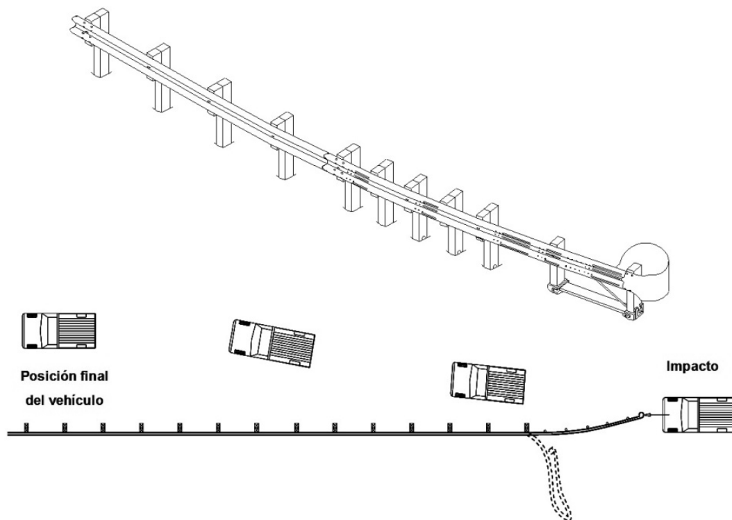
FIGURA 27.- Sección de amortiguamiento redireccionable-traspasable (OD-4.4.1/RT) en barrera de orilla de corona no paralela al arroyo vial (OD-4.1.2)
