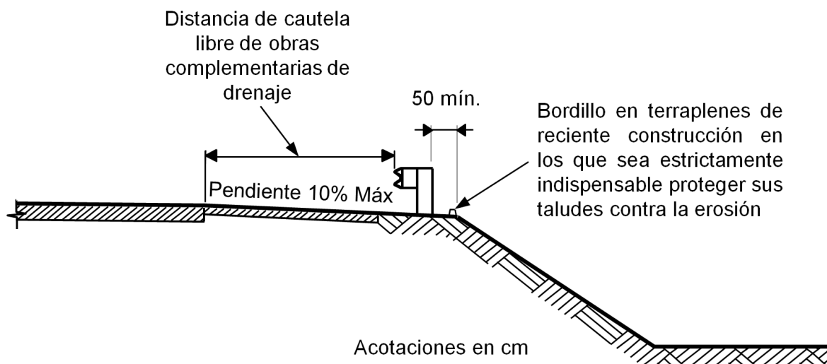
FIGURA 7.- Pendiente transversal dentro de la distancia de cautela
