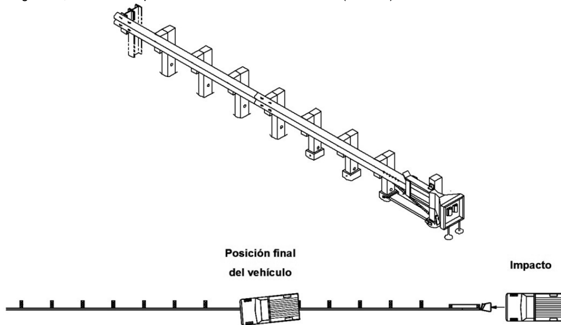
FIGURA 25.- Sección de amortiguamiento redireccionable- no traspasable (OD-4.4.1/RNT) en barrera de orilla de corona paralela al arroyo vial (OD-4.1.1 y OD-4.1.2)
