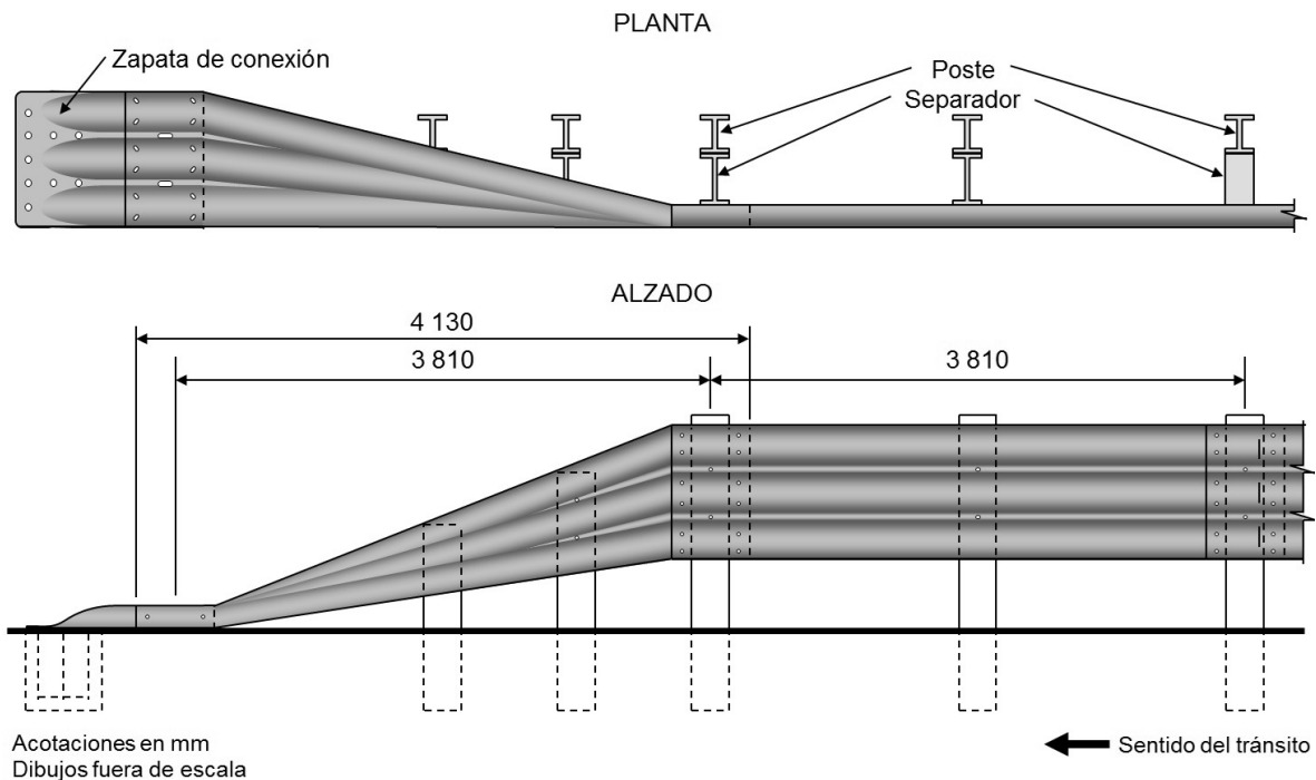
FIGURA 29.- Sección terminal aterrizada para vigas acanaladas de dos y de tres crestas (OD-4.4.2/A)
