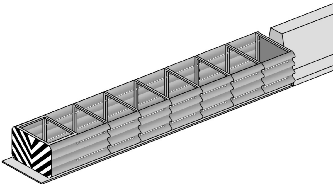
FIGURA 26.- Sección de amortiguamiento redireccionable- no traspasable (OD-4.4.1/RNT) en barrera separadora de sentidos de circulación (OD-4.2.)
