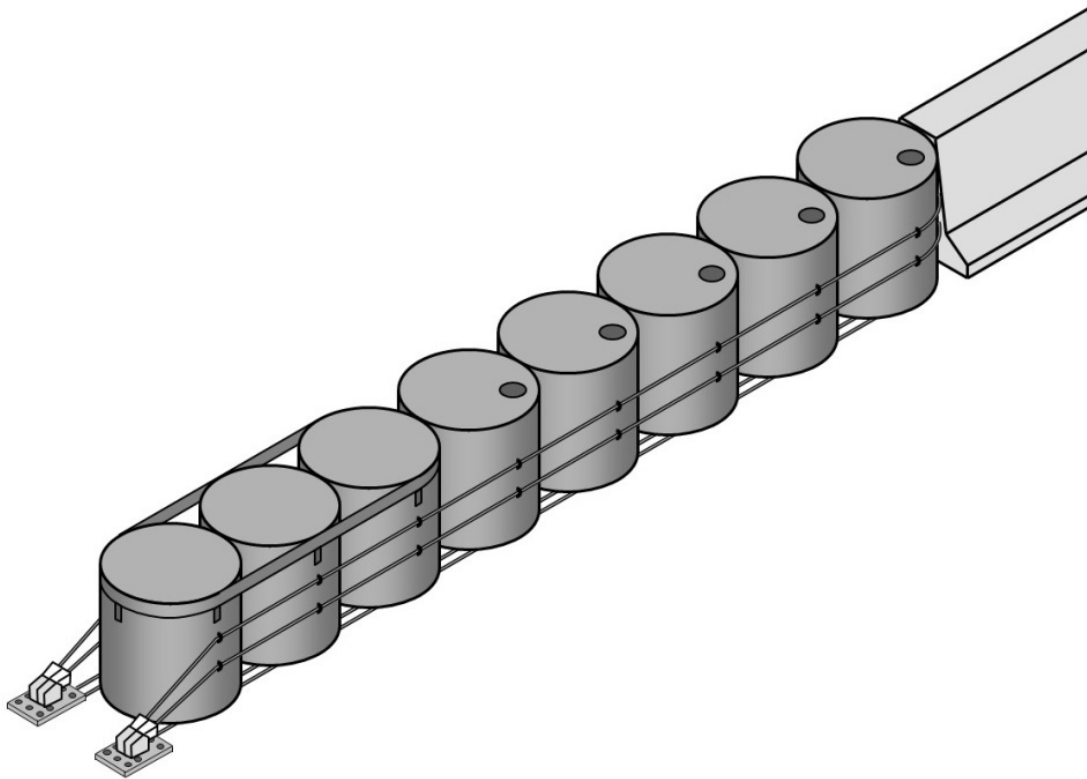
FIGURA 24.- Sección de amortiguamiento no redireccionable (OD-4.4.1/NR)
