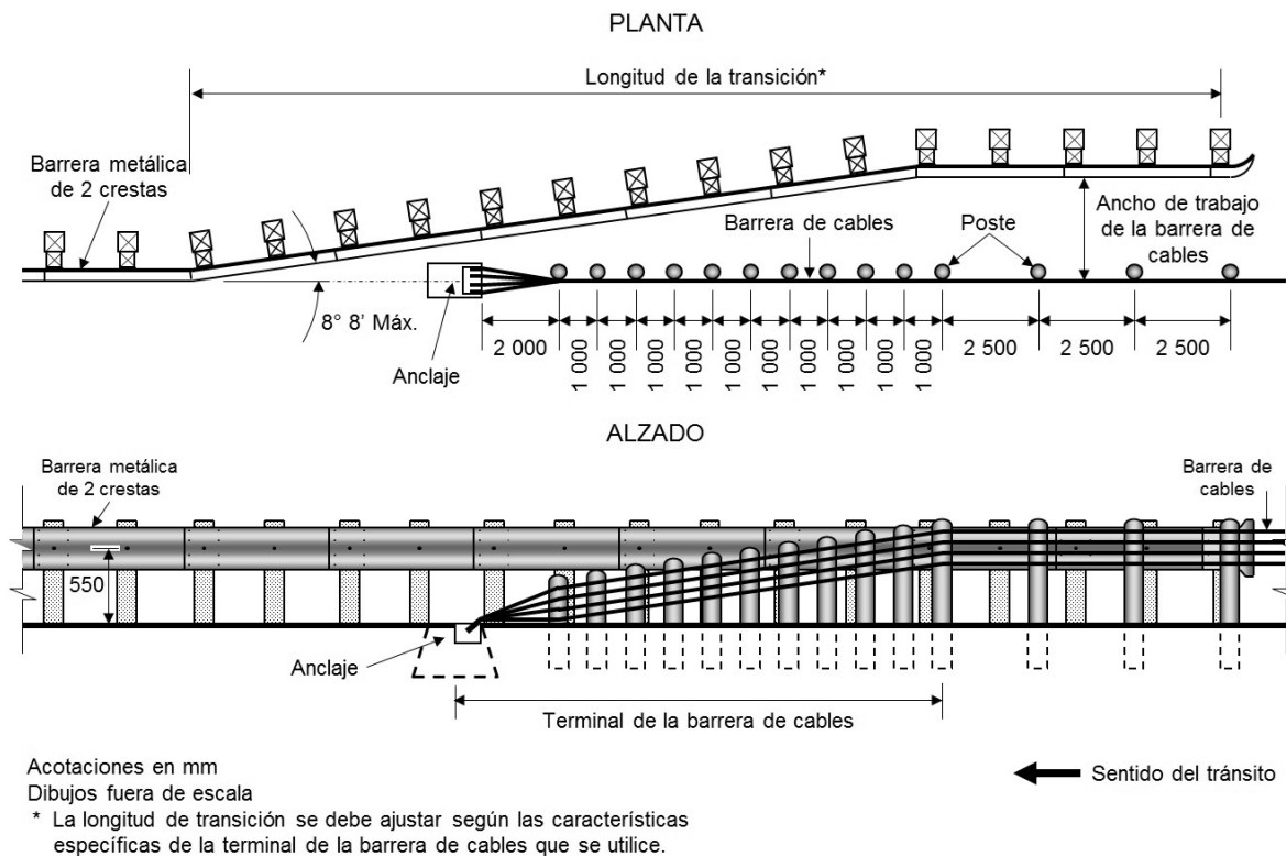
FIGURA 23.- Transición de barrera flexible de cables de acero
