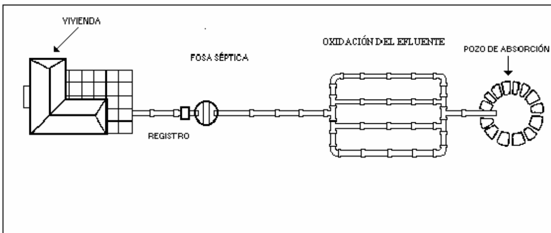
FIGURA 1. SISTEMA DE TRATAMIENTO FOSEA SEPTICA (figura ilustrativa)
