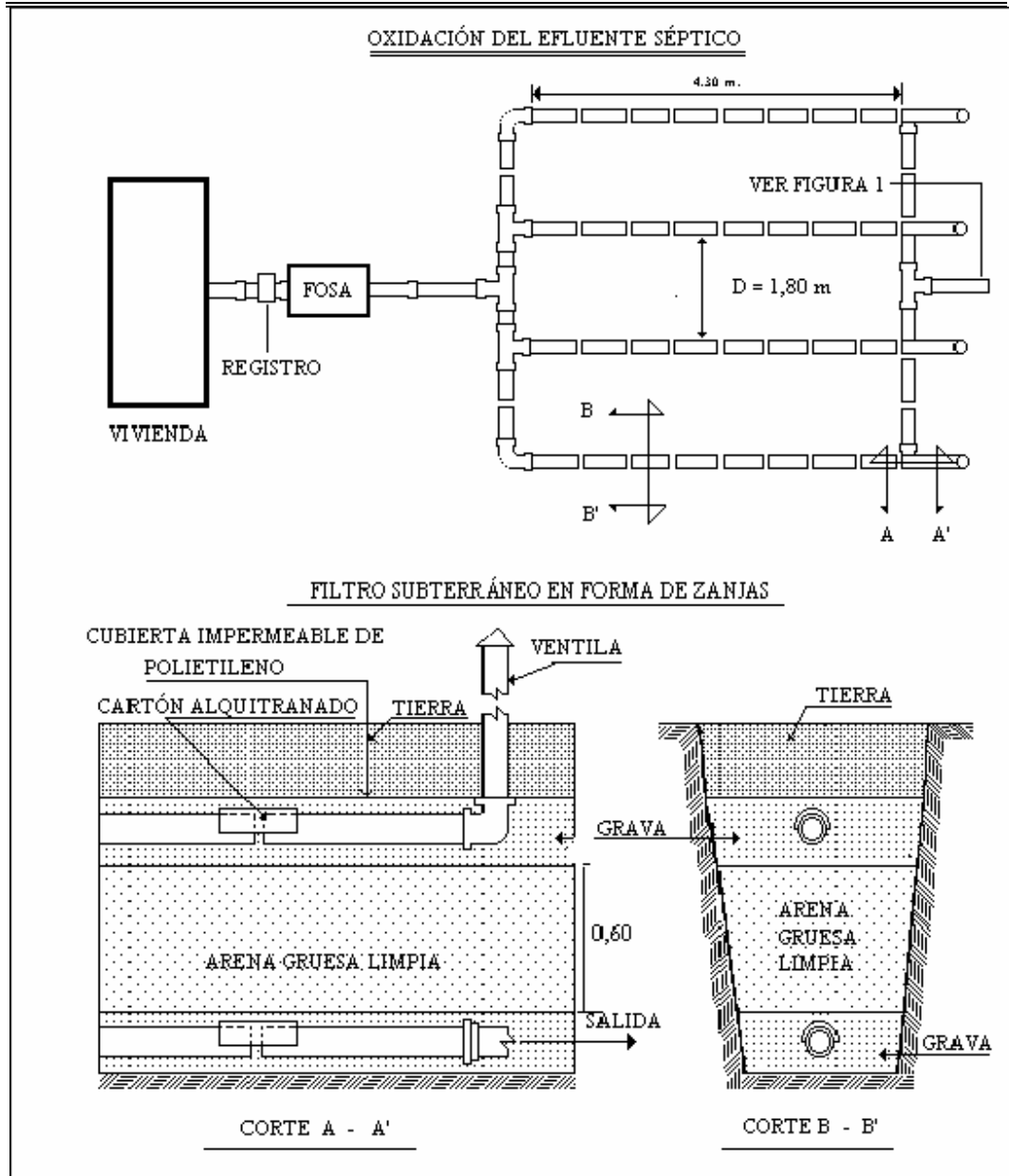
FIGURA 8. FILTROS SUBTERRÁNEOS DE ARENA (figura ilustrativa)
