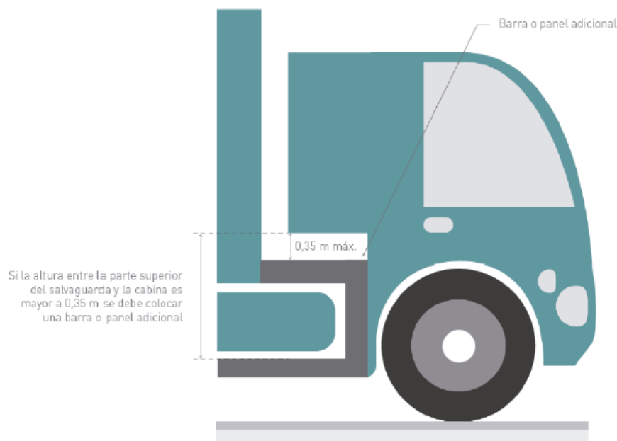
Figura 4. Forma del salvaguarda en la parte frontal cuando existe espacio con la ca
