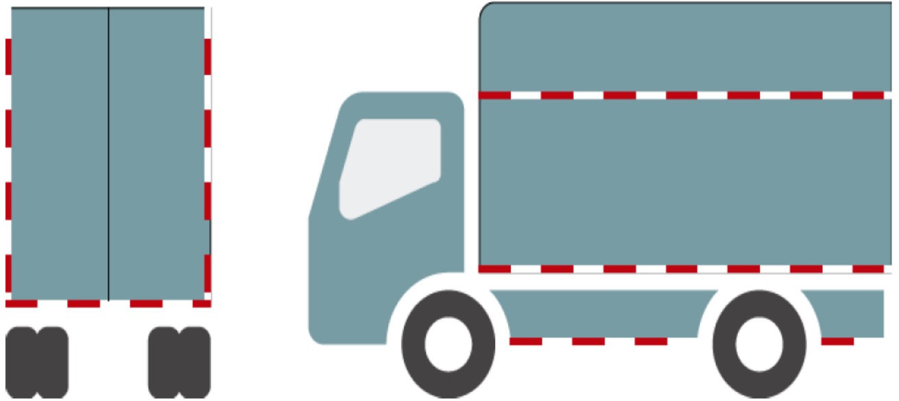
Figura 5. Ejemplo de colocación de cintas reflejantes en vehículos de carga
